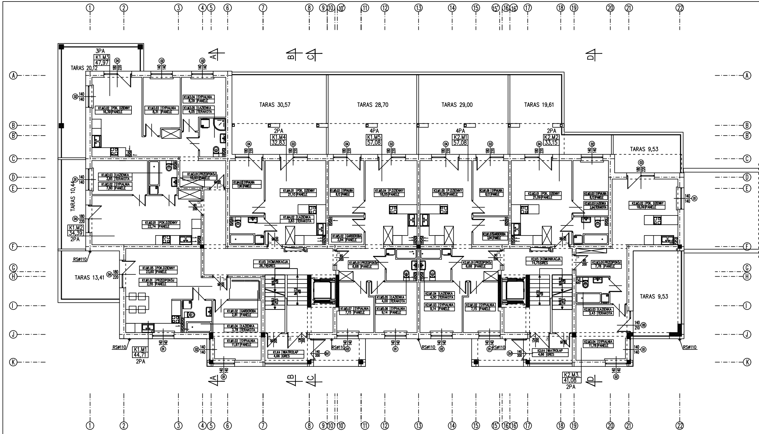
RZUT PARTERU SKALA 1:100
