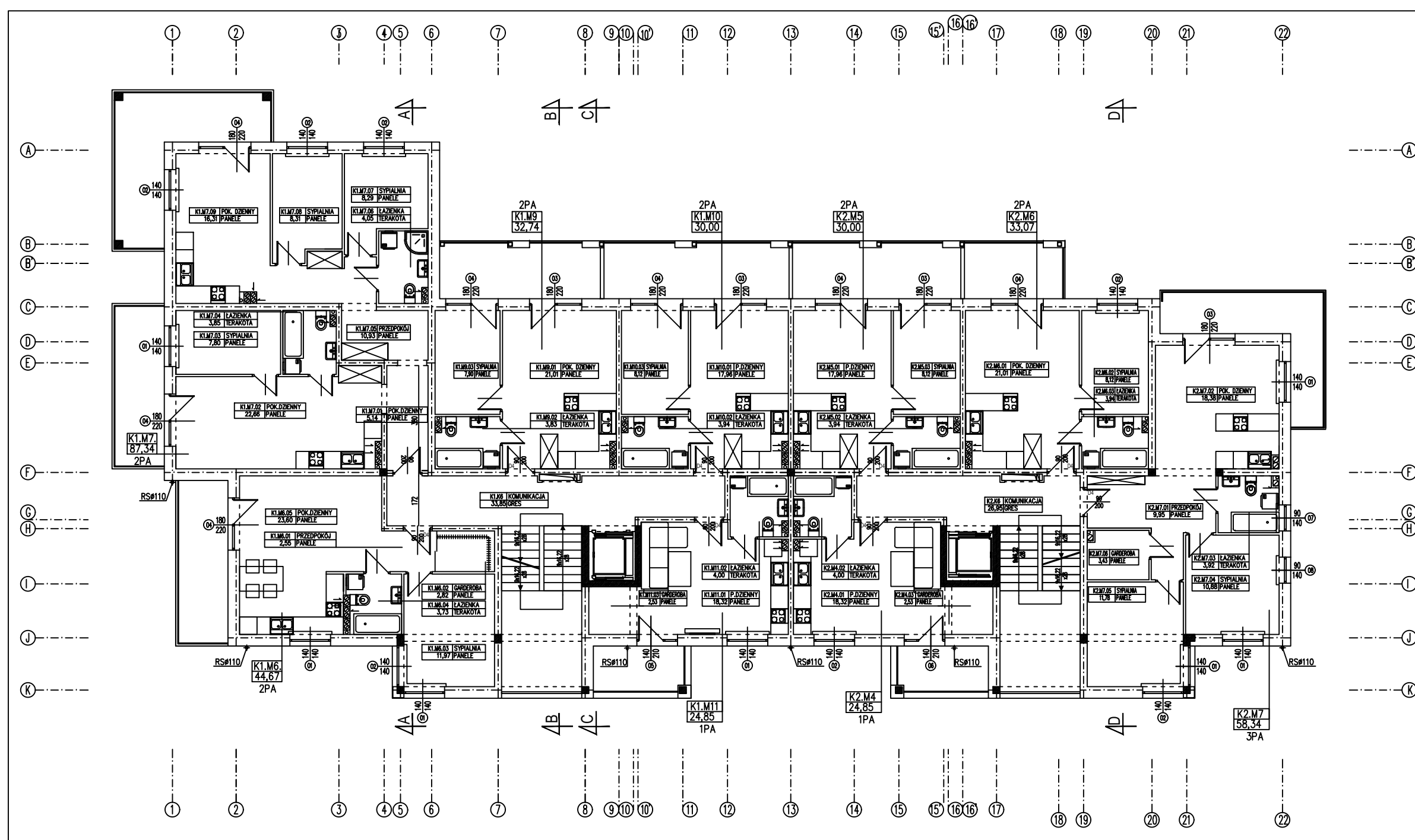
RZUT I PIĘTRA SKALA 1:100
